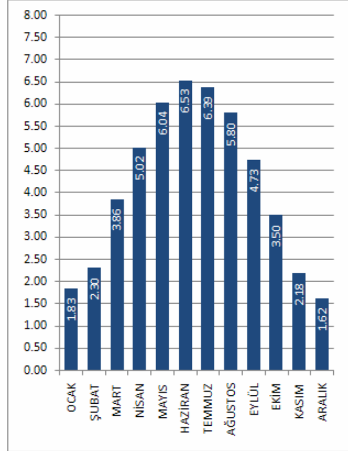
EGE BÖLGESİ GLOBAL RADYASYON DEĞERLERİ (KWh/m 2 -gün)
