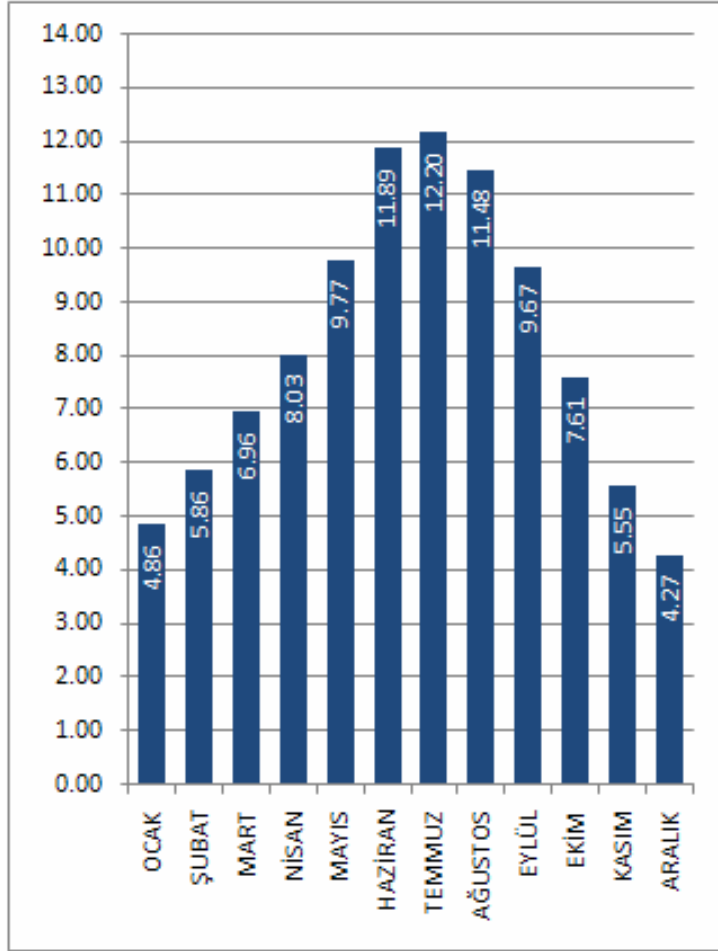
İZMİR İLİ GÜNEŞLENME SÜRESİ DEĞERLERİ (Saat)
