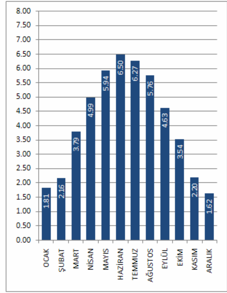
İZMİR İLİ GLOBAL RADYASYON DEĞERLERİ (KWh/m 2 -gün)
