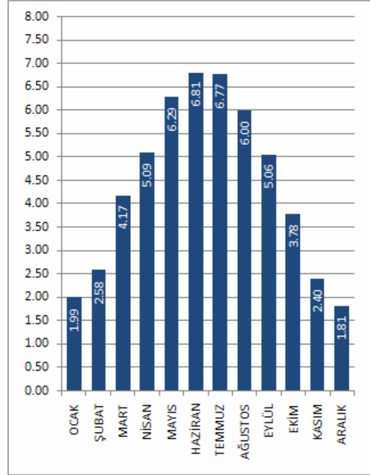
K.MARAŞ İLİ GLOBAL RADYASYON DEĞERLERİ (KWh/m 2 -gün)
