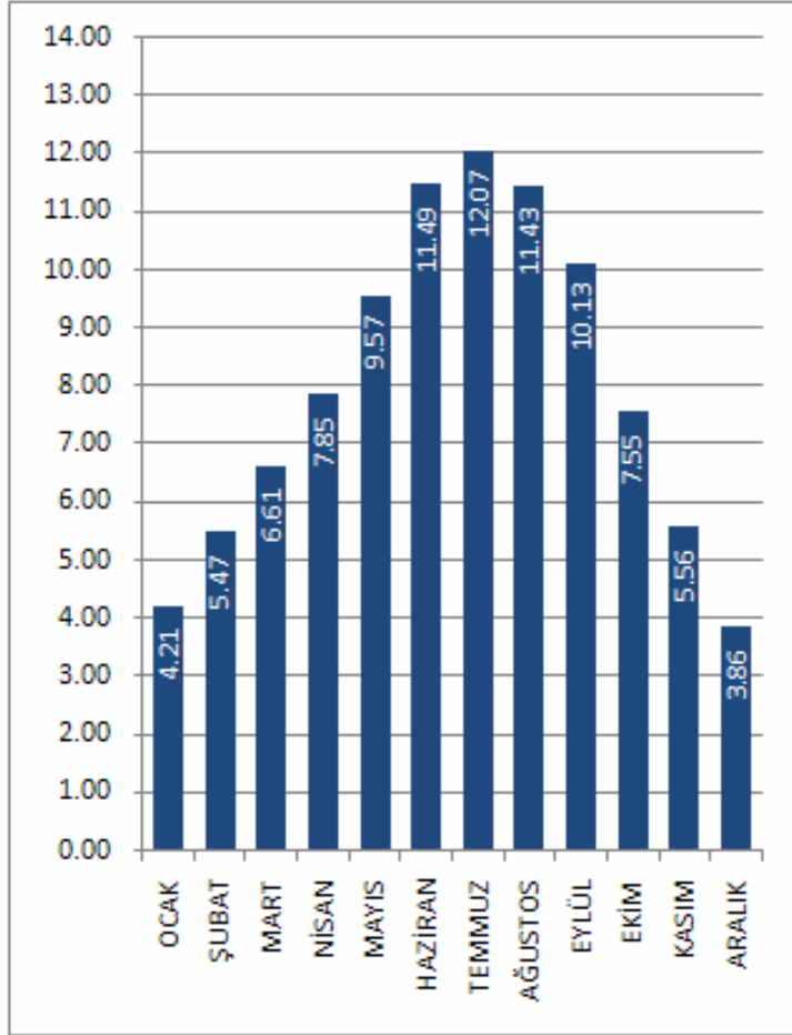
K.MARAŞ İLİ GÜNEŞLENME SÜRESİ DEĞERLERİ (Saat)
