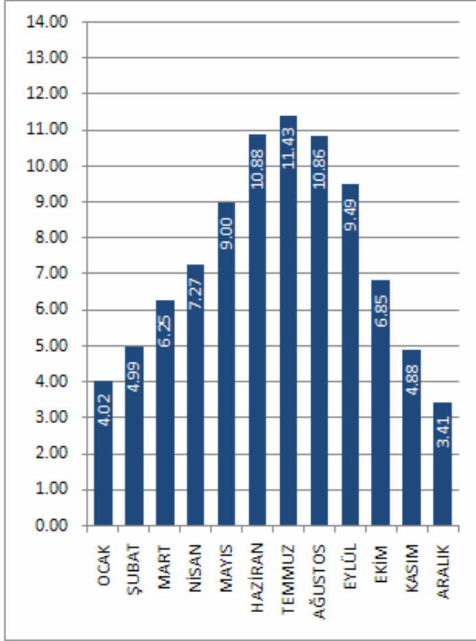
TUNCELİ İLİ GÜNEŞLENME SÜRESİ DEĞERLERİ (Saat)
