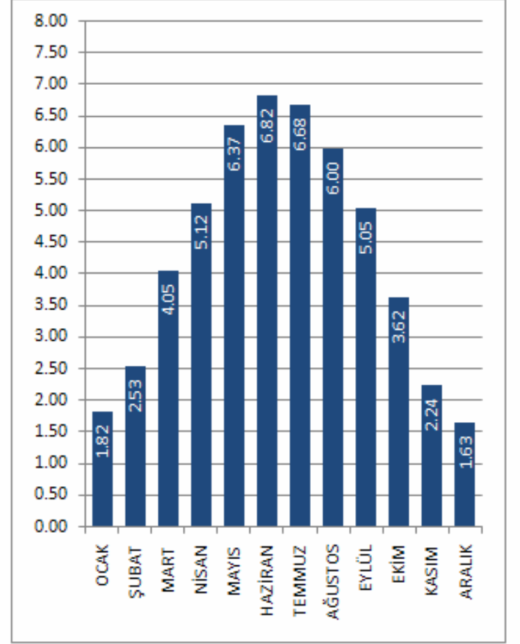
TUNCELİ İLİ GLOBAL RADYASYON DEĞERLERİ (KWh/m 2 -gün)
